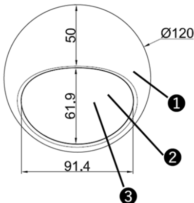
(ボックス正面寸法)
