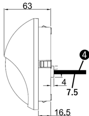
(灯具横面寸法)
