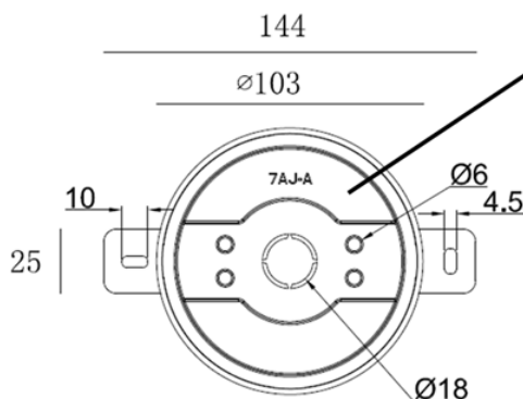
(ボックス正面寸法)
